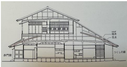
図3 成巽閣の構造(パンフレットによる)
