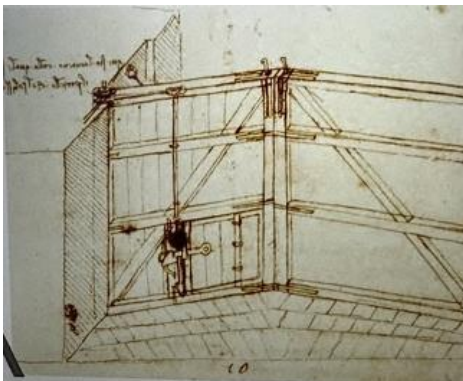
図2 ダ・ヴィンチがデッサンした閘門
