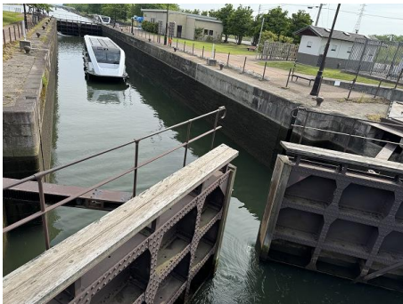
写真4 下流側から眺めた中島閘門
