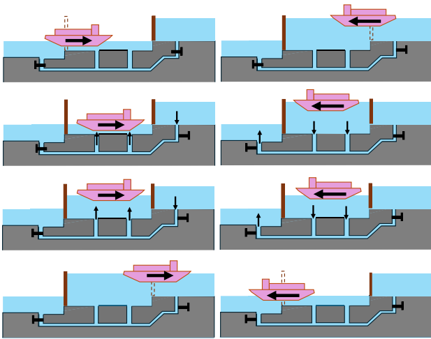
図1 中島閘門の仕組み(著者による)
